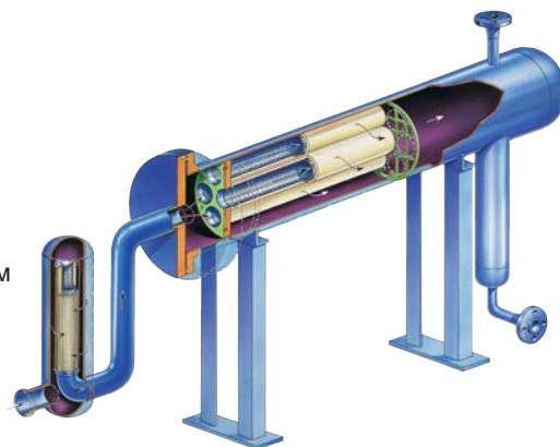
Горизонтальная конфигурация коалесцера Палл для жидких эмульсий Конфигурация с предфильтром слева и коалесцером Аквасеп Плюс/Фейзсеп справа. Свободная от загрязнений сплошная фаза выходит сверху справа, удаленная фаза выходит внизу справа.
