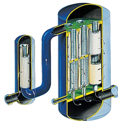
Вертикальная конфигурация коалесцера Палл для жидких эмульсий Конфигурация с предфильтром слева и коалесцером Аквасеп Плюс/Фейзсеп справа. Вода выходит внизу налево, свободный от воды продукт внизу направо.
