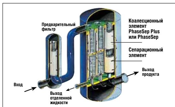
Система сепарации жидкостей с коалесцирующими фильтроэлементами AquaSep Plus/PhaseSep и сепарационными элементами в вертикальном корпусе.
