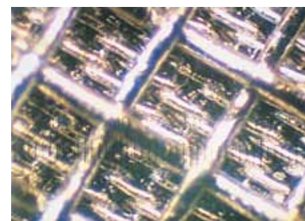
Rigimesh – приблизительная объемная пористость = 30 %.
