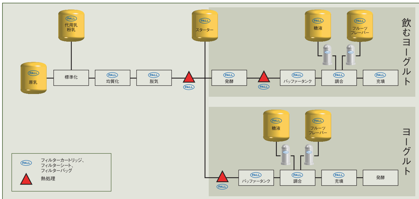
図2 一般的なヨーグルト製造工程
