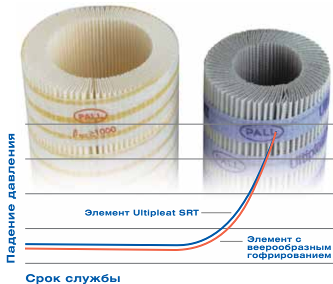
Рисунок 4: Кривая срока службы показывает, что элемент Ultipleet SRT и более крупный элемент с традиционным гофрированием могут иметь одинаковый срок службы
