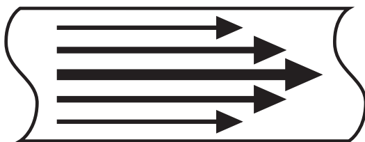
Régime laminaire
