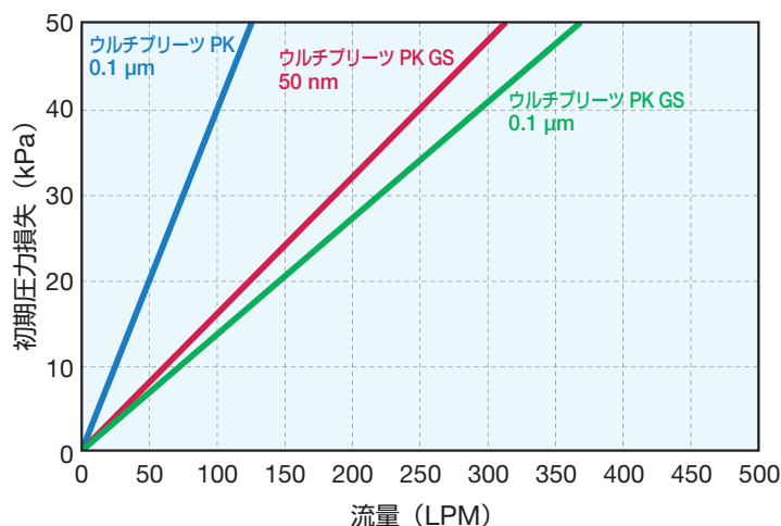
図1: UPK510GSカートリッジの流量特性比較
